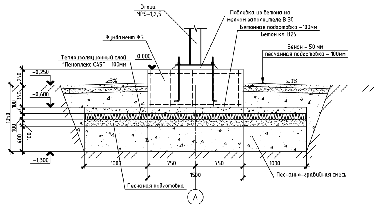
Схема установки фундамента Ф5
