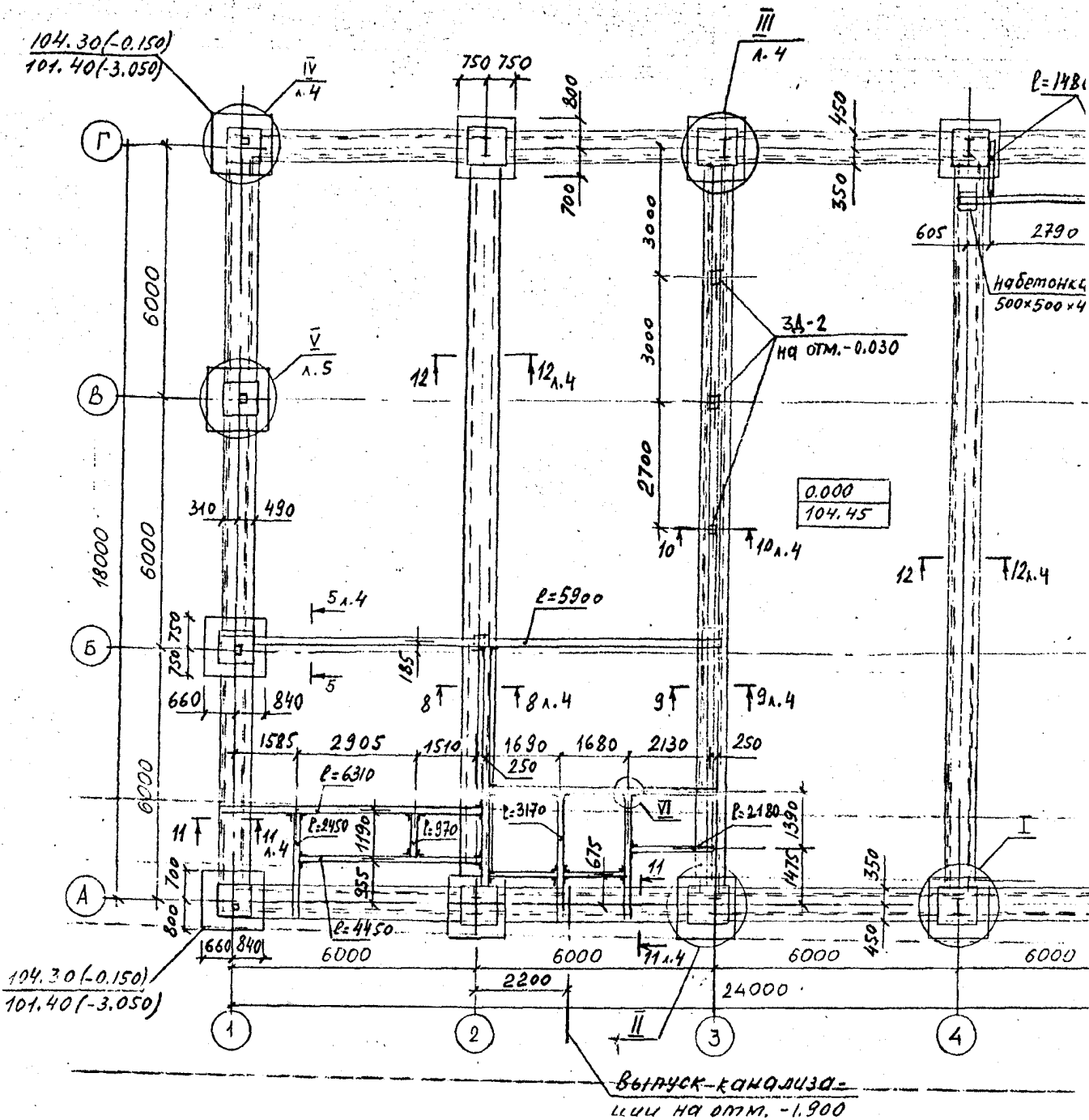
Схема расположения фундаментов М 1:100
